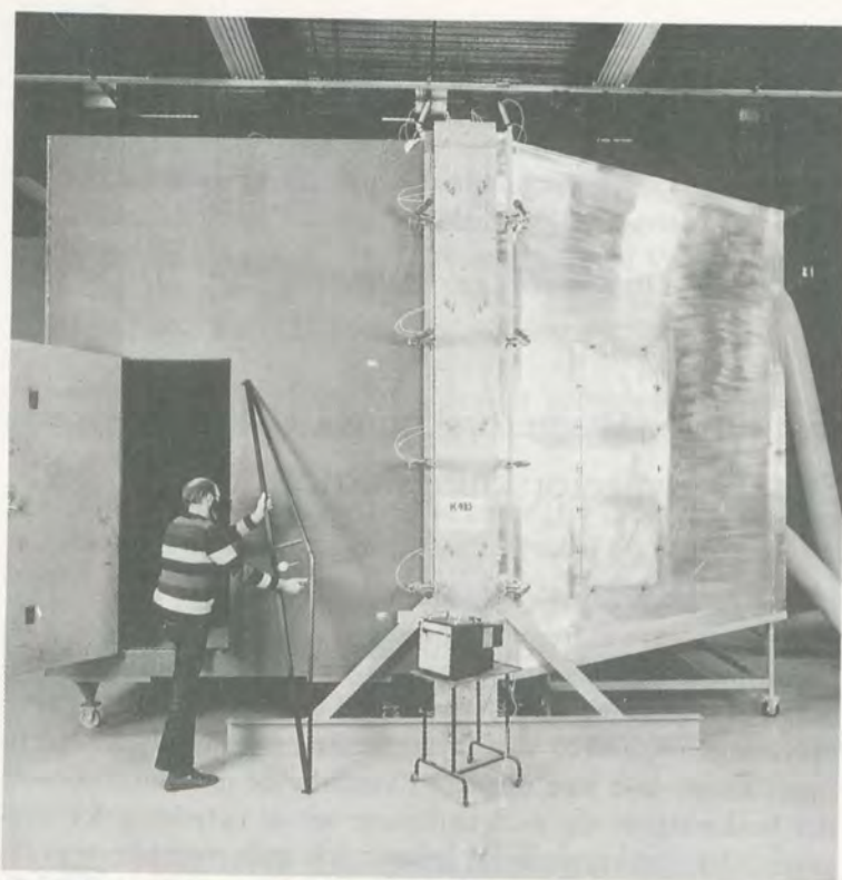
Statens Byggeforskningsinstitut tilbød virksomheder afprøvning af alle slags byggematerialer og havde dertil udviklet en lang række maskiner ofte af besynderligt udseende. Her ses "Varm/kold kassen" - et klimaapparat til undersøgelse af, hvordan byggekomponenter opfører sig under varierende fugt- og temperaturforhold. Billedet er fra 1989 (Statens Byggeforskningsinstitut).
