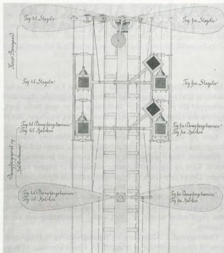
DSB har afleveret en række tegningssamlinger til Rigsarkivet. Heri indgår bl.a. denne afbildning af en optisk telegraf for Korsør Banegård tegnet i 1883 (Rigsarkivet: Kort og tegninger, DSB, Baneafd., Ældre Normaltegninger M. VI a nr. 22).
